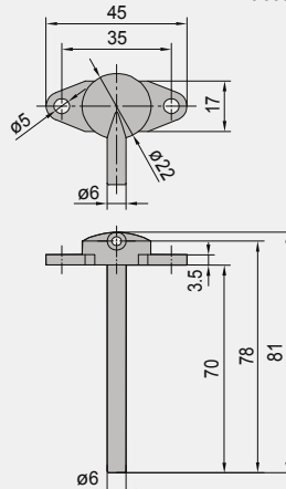
ASD - 07 embouts de raccordement
